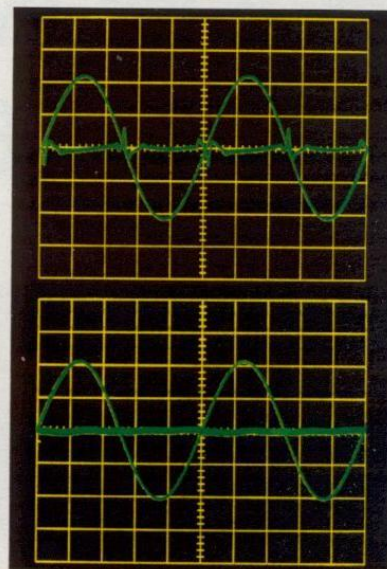
Class B Verstärker-Ausgang-Wellenform und Verzerrungs-Wellenform (20 kHz).
